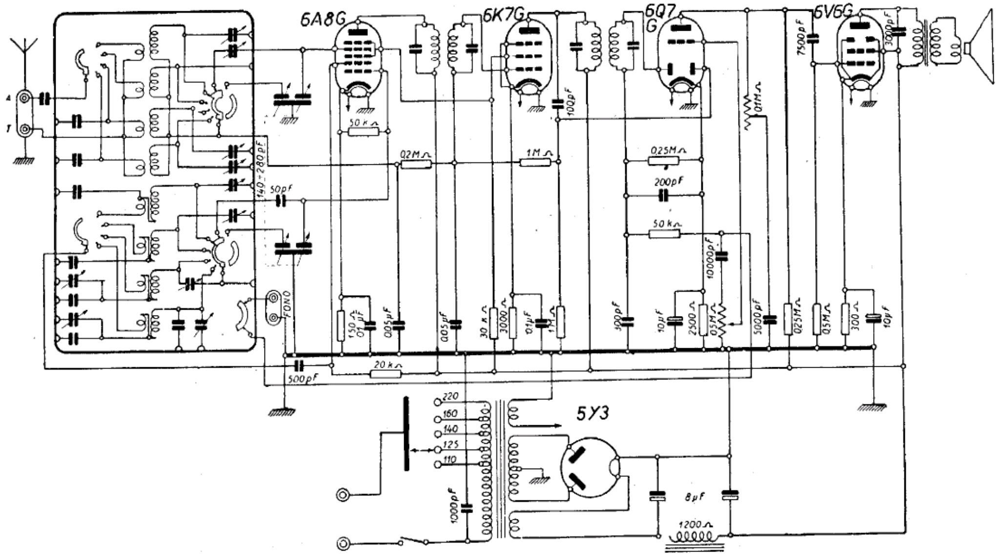
VARA RADIO - Mod. 604 e mod. 605 - Quattro gamme. Media frequenza 467 kc/s. Sensibilità media 30 microvolt. Potenza d'uscita 3,5 W. Consumo 60 W.
